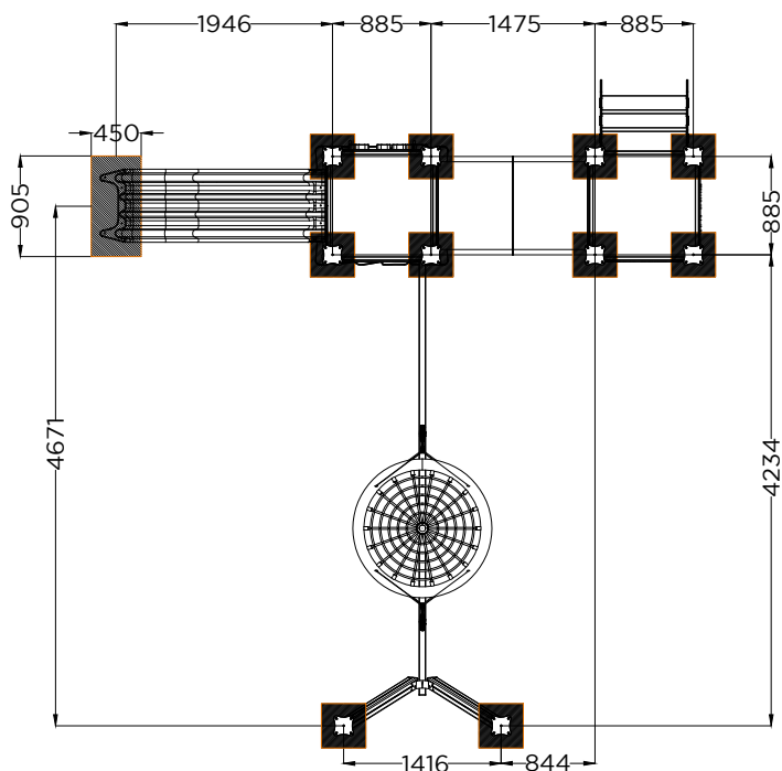
PLANTA . ESQUEMA DE FIXAÇÃO PLAN . INSTALLATION PLAN
