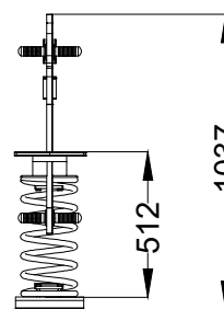
ALÇADO FRONTAL FRONT VIEW
