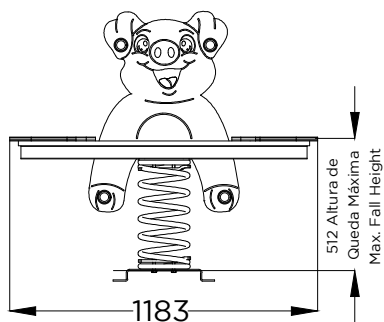
ALÇADO LATERAL SIDE VIEW
