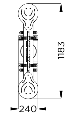
PLANTA PLAN
