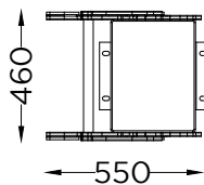
PLANTA PLAN
