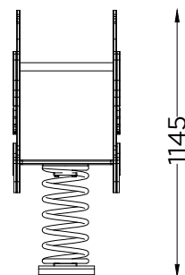
ALÇADO FRONTAL FRONT VIEW
