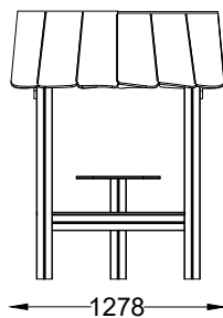
ALÇADO LATERAL SIDE VIEW
