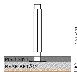
BASE BETÃO + PISO SINTÉTICO
