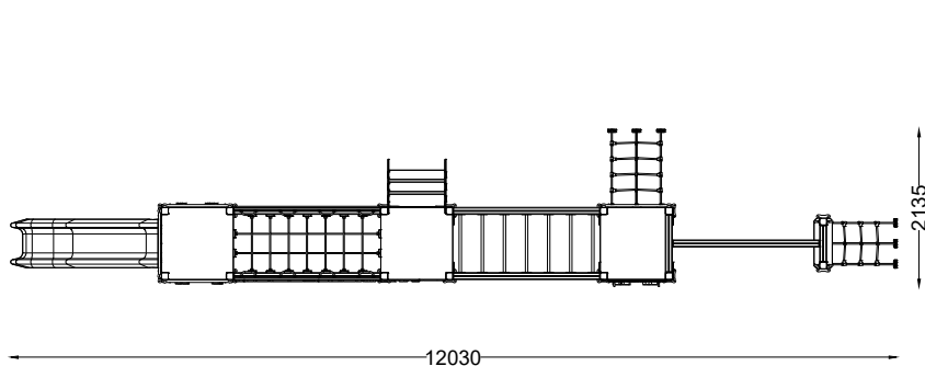
PLANTA - ESPAÇO DE SEGURANÇA NECESSÁRIO PLAN - SAFETY SPACE REQUIRED
