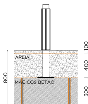
MACIÇOS BETÃO + PISO AREIA
