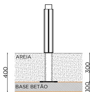
BASE BETÃO + PISO AREIA
