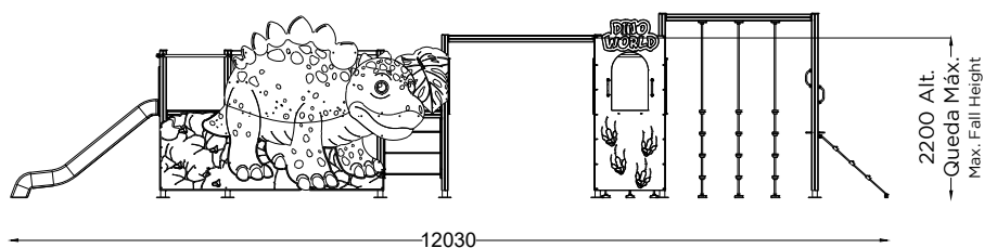
ALÇADO LATERAL SIDE VIEW
