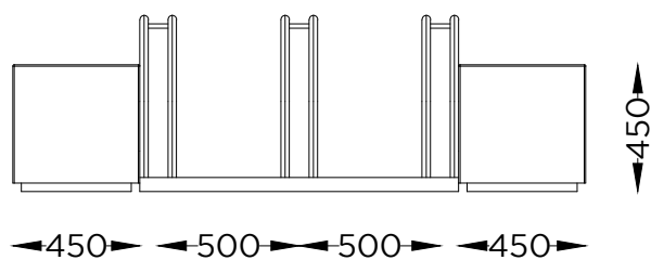
ALÇADO FRONTAL FRONT VIEW
