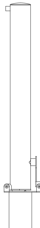
ALÇADO FRONTAL FRONT VIEW
