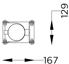
PLANTA PLAN
