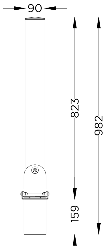
ALÇADO LATERAL SIDE VIEW
