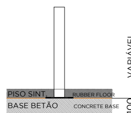
BASE BETÃO + PISO SINTÉTICO CONCRETE BASE + RUBBER FLOOR
