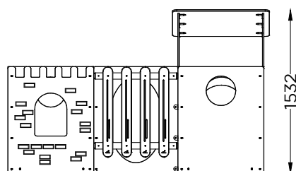
ALÇADO FRONTAL FRONT VIEW
