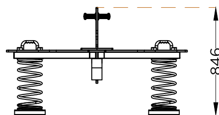
ALÇADO LATERAL SIDE VIEW
