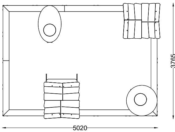
PLANTA PLAN
