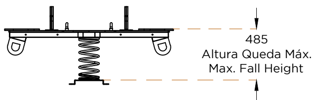
ALÇADO FRONTAL FRONT VIEW
