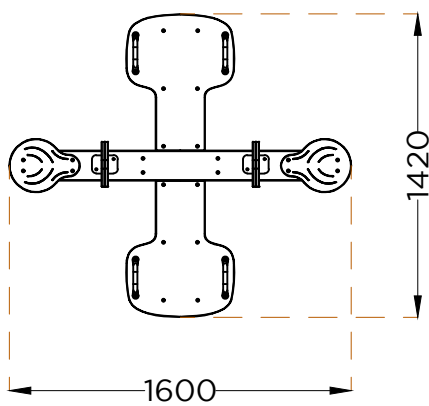
PLANTA PLAN
