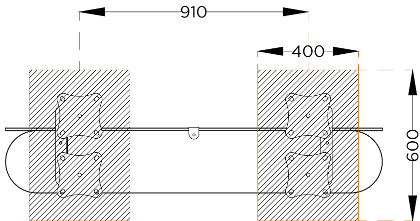
PLANTA . ESQUEMA DE FIXAÇÃO PLAN . INSTALLATION PLAN
