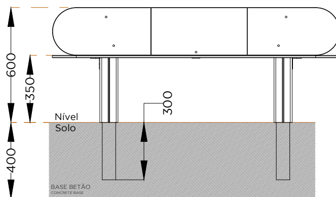
ALÇADO . ESQUEMA DE FIXAÇÃO POR ENTERRAMENTO SIDE VIEW . DIRECT BURIAL MOUNTING
