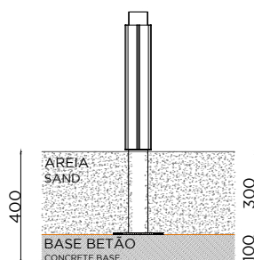
ALÇADO . ESQUEMA DE FIXAÇÃO POR ENTERRAMENTO SIDE VIEW . DIRECT BURIAL MOUNTING
