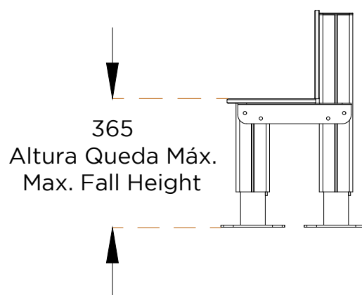
ALÇADO FRONTAL FRONT VIEW
