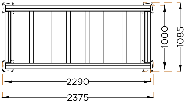
PLANTA PLAN
