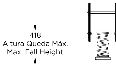
ALÇADO LATERAL SIDE VIEW
