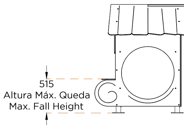
ALÇADO LATERAL SIDE VIEW
