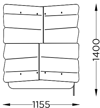
PLANTA PLAN
