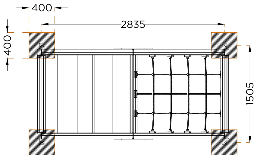
PLANTA . ESQUEMA DE FIXAÇÃO PLAN . INSTALLATION PLAN
