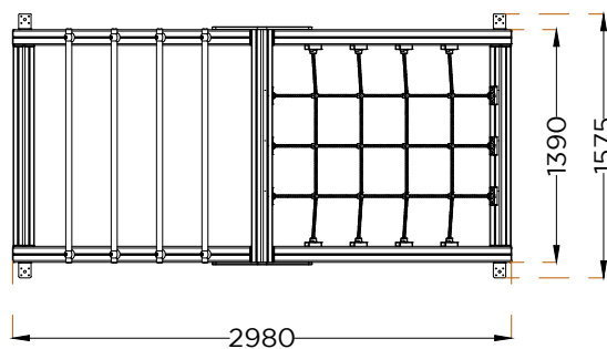
PLANTA PLAN
