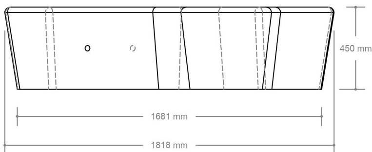
Alçado Lateral Lateral View
