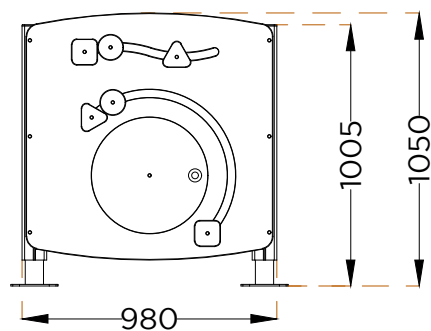
ALÇADO FRONTAL FRONT VIEW
