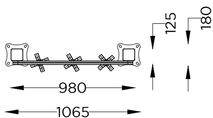
PLANTA PLAN
