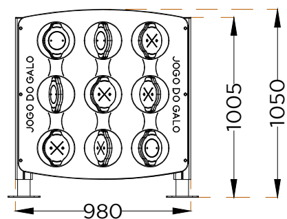
ALÇADO FRONTAL FRONT VIEW
