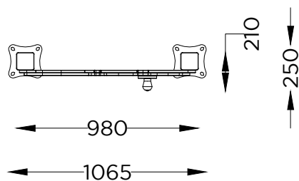
PLANTA PLAN
