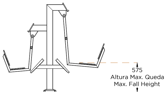
ALÇADO FRONTAL FRONT VIEW
