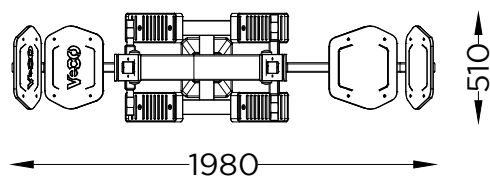
PLANTA PLAN
