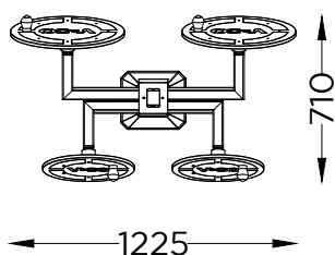
PLANTA PLAN
