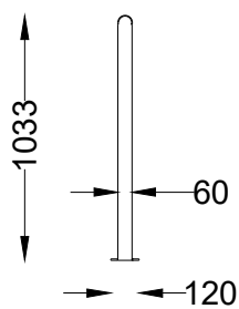
ALÇADO LATERAL SIDE VIEW
