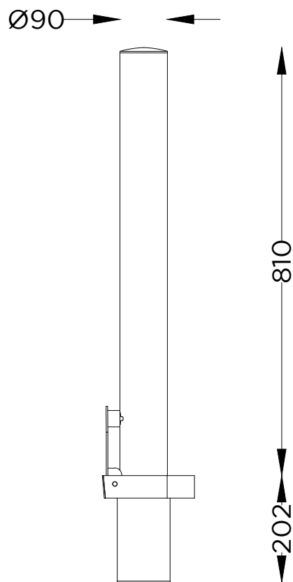
ALÇADO LATERAL SIDE VIEW
