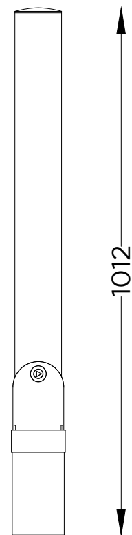
ALÇADO FRONTAL FRONT VIEW
