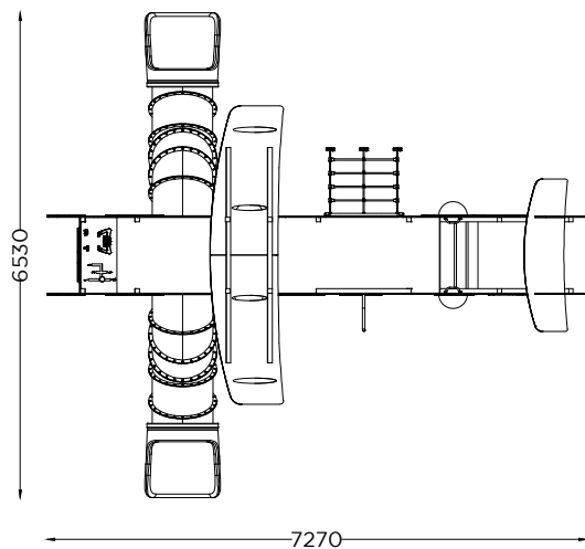
PLANTA PLAN
