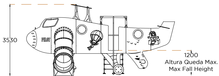
ALÇADO LATERAL SIDE VIEW
