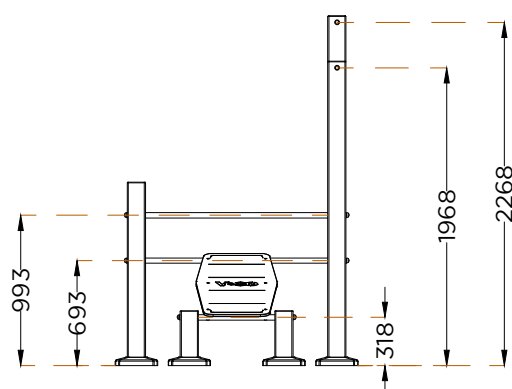
ALÇADO LATERAL SIDE VIEW
