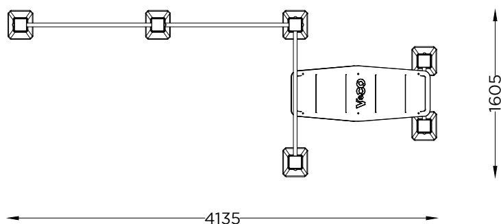
PLANTA PLAN
