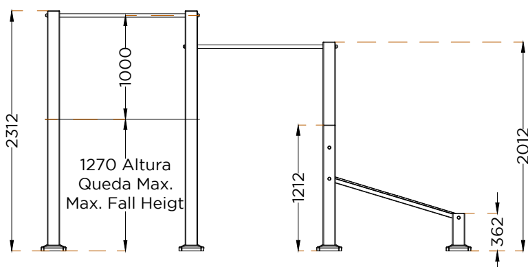
ALÇADO FRONTAL FRONT VIEW
