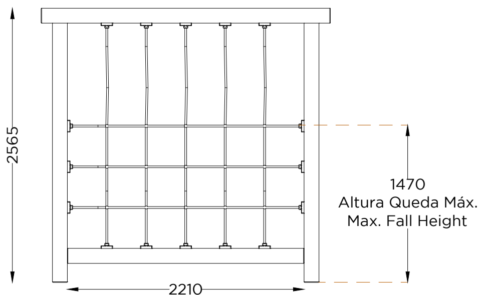
ALÇADO FRONTAL FRONT VIEW
