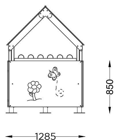
ALÇADO FRONTAL FRONT VIEW
