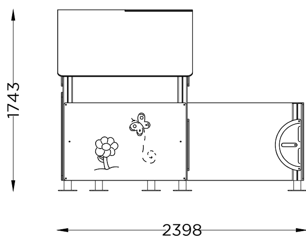
ALÇADO LATERAL SIDE VIEW
