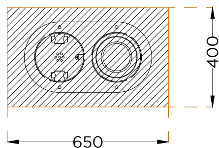
PLANTA . ESQUEMA DE FIXAÇÃO PLAN . INSTALLATION PLAN
