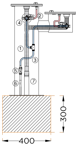
ALÇADO FRONTAL FRONT VIEW
