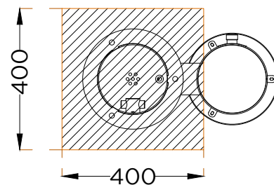
PLANTA . ESQUEMA DE FIXAÇÃO PLAN . INSTALLATION PLAN
