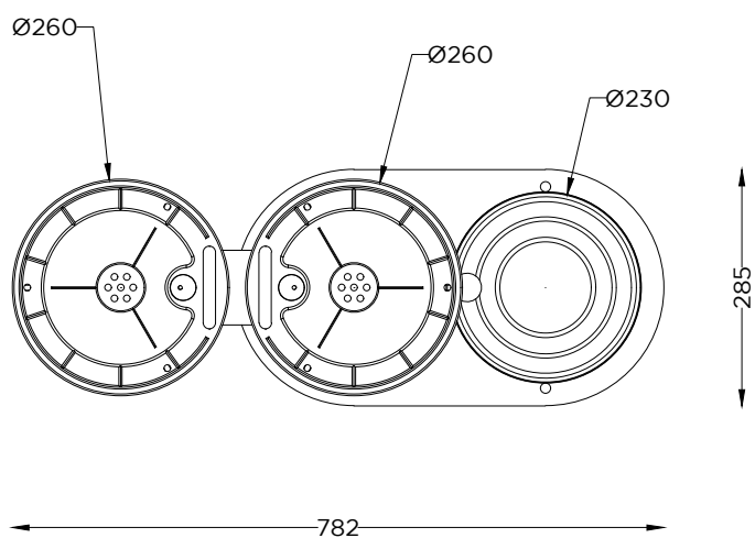
PLANTA PLAN
