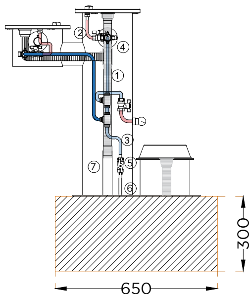
ALÇADO FRONTAL FRONT VIEW
