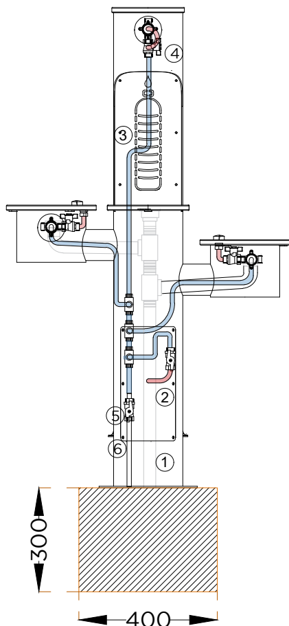
ALÇADO FRONTAL FRONT VIEW
