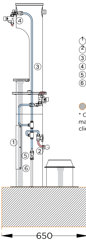
ALÇADO LATERAL SIDE VIEW
