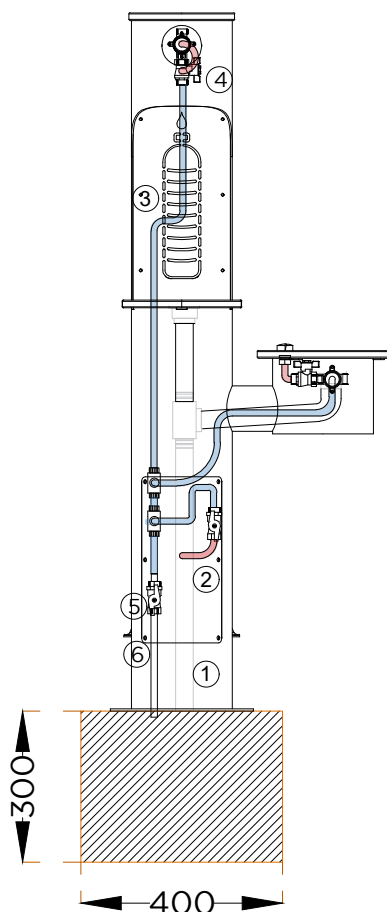
ALÇADO FRONTAL FRONT VIEW
