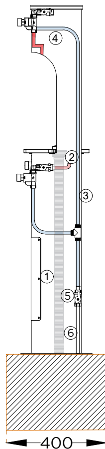
ALÇADO LATERAL SIDE VIEW
