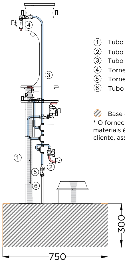
ALÇADO LATERAL SIDE VIEW
