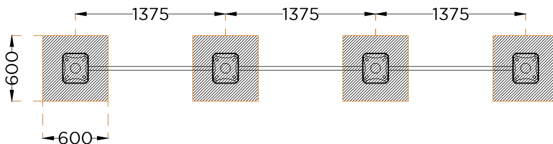
PLANTA . ESQUEMA DE FIXAÇÃO PLAN . INSTALLATION PLAN
