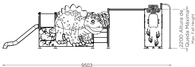
ALÇADO LATERAL SIDE VIEW
