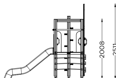
ALÇADO FRONTAL FRONT VIEW
