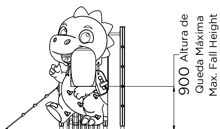
ALÇADO LATERAL SIDE VIEW
