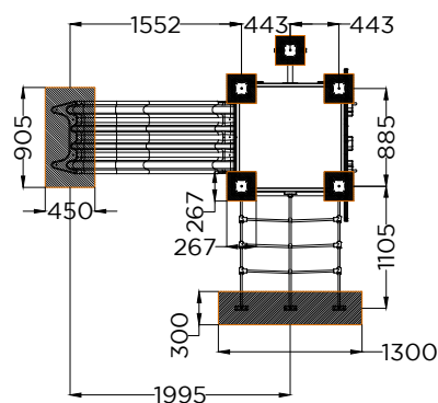
PLANTA . ESQUEMA DE FIXAÇÃO PLAN . INSTALLATION PLAN
