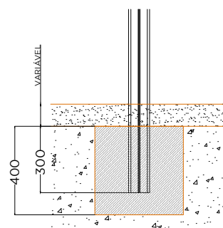
FIXAÇÃO POR CHUMBAMENTO BURIAL
