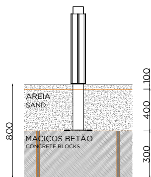
MACIÇOS BETÃO + PISO AREIA CONCRETE BLOCKS + SAND LAYER
