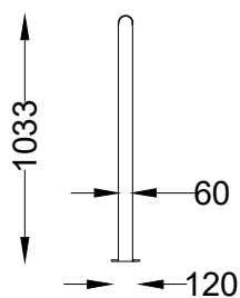
ALÇADO LATERAL SIDE VIEW
