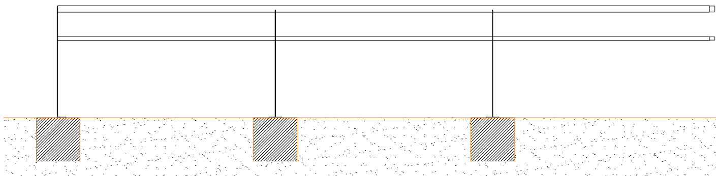
ALÇADO FRONTAL . ESQUEMA DE FIXAÇÃO FRONT VIEW . INSTALLATION PLAN
