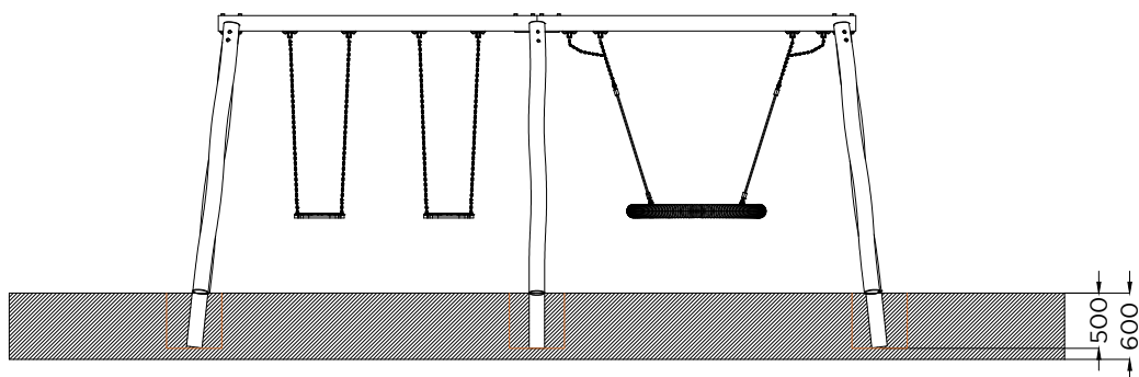
ALÇADO . ESQUEMA DE FIXAÇÃO SIDE VIEW . INSTALLATION PLAN
