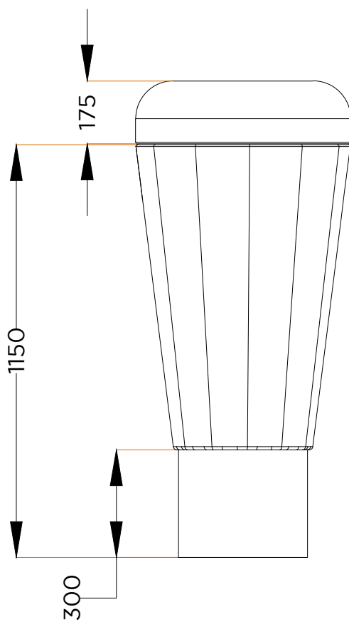
ALÇADO LATERAL SIDE VIEW
