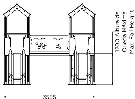
ALÇADO FRONTAL FRONT VIEW
