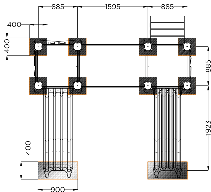
PLANTA . ESQUEMA DE FIXAÇÃO PLAN . INSTALLATION PLAN
