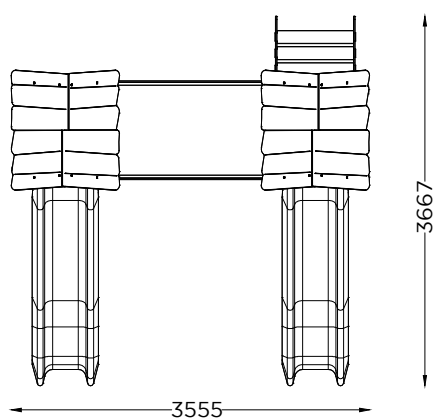
PLANTA PLAN
