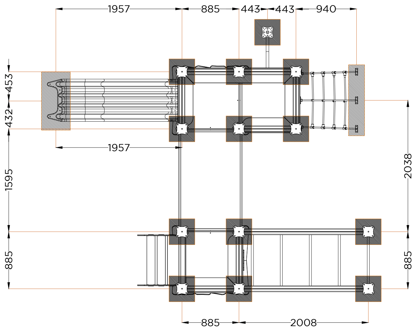
PLANTA . ESQUEMA DE FIXAÇÃO PLAN . INSTALLATION PLAN
