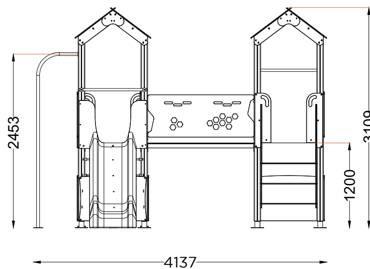
ALÇADO LATERAL SIDE VIEW
