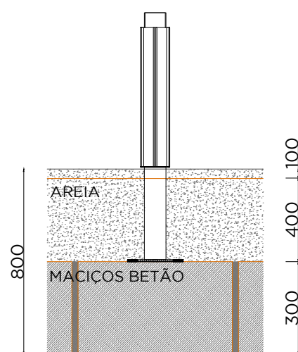
MACIÇO BETÃO + PISO AREIA
