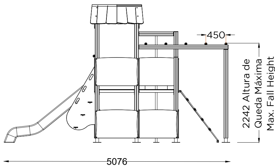
ALÇADO FRONTAL FRONT VIEW
