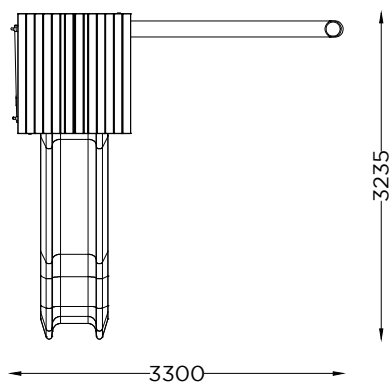
PLANTA PLAN
