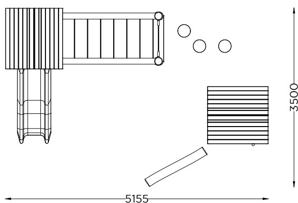
PLANTA PLAN
