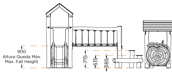
ALÇADO FRONTAL FRONT VIEW
