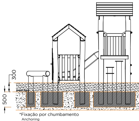
ALÇADOS . ESQUEMAS DE FIXAÇÃO SIDE VIEW . INSTALLATION PLAN
