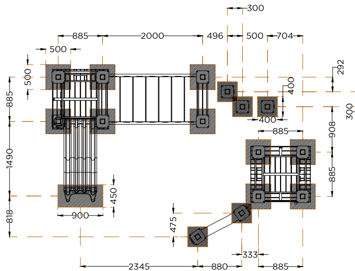
PLANTA . ESQUEMA DE FIXAÇÃO PLAN . INSTALLATION PLAN
