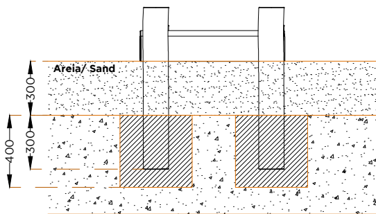
ALÇADOS . ESQUEMA DE FIXAÇÃO SIDE VIEW . INSTALLATION PLAN
