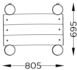
PLANTA PLAN
