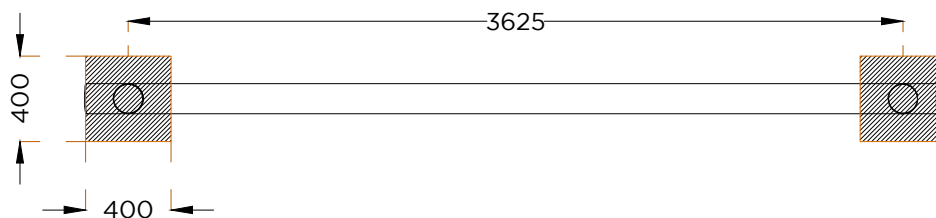
PLANTA . ESQUEMA DE FIXAÇÃO PLAN . INSTALLATION PLAN
