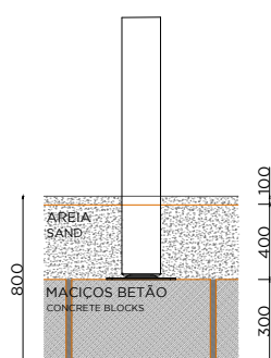
MACIÇOS BETÃO + PISO AREIA CONCRETE BLOCK + SAND LAYER
