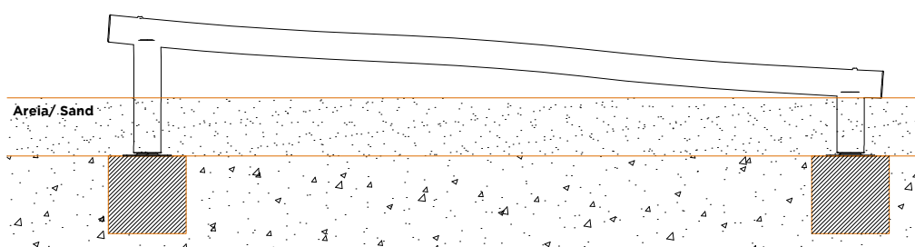
*Fixação por sapata metálica Metal shoe
