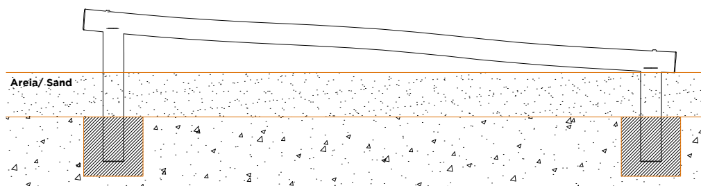
*Fixação enterramento Burial
