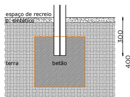
ESQUEMA DE FIXAÇÃO POR ENTERRAMENTO
