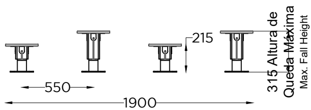
ALÇADO LATERAL SIDE VIEW
