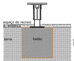
ESQUEMA DE FIXAÇÃO POR SAPATA
