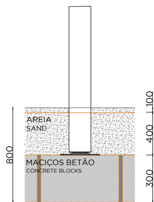
MACIÇOS BETÃO + PISO AREIA CONCRETE BLOCK + SAND LAYER
