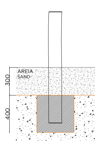
MACIÇO BETÃO + PISO AREIA CONCRETE BLOCK + SAND LAYER
