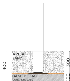
BASE BETÃO + PISO AREIA CONCRETE BASE + SAND LAYER
