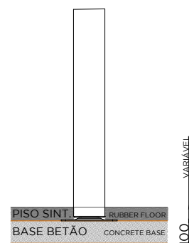
BASE BETÃO + PISO SINTÉTICO CONCRETE BASE + RUBBER FLOOR
